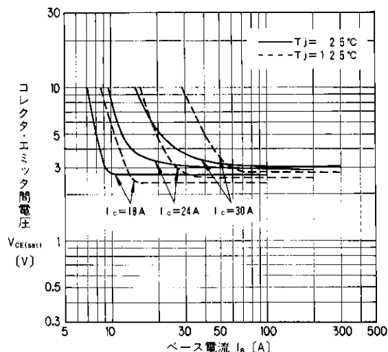
出力特性
