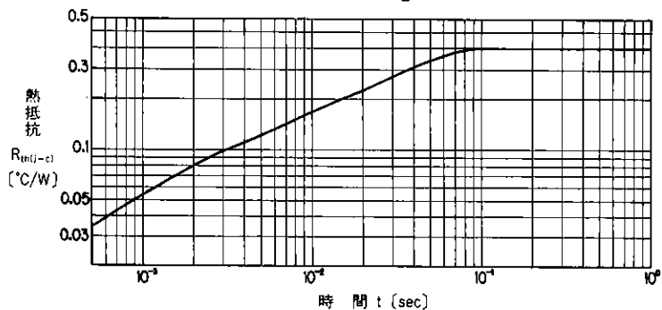
過渡熱抵抗(トランジスタ)特性
