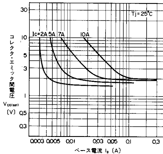
出力特性
