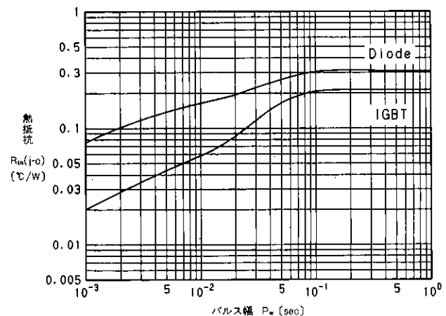
過渡熱抵抗特性 Transient Thermal Resistance
