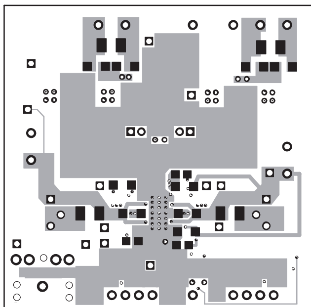
Figure 3–28. TPA005D14 Class-D EVM Bottom Layer
