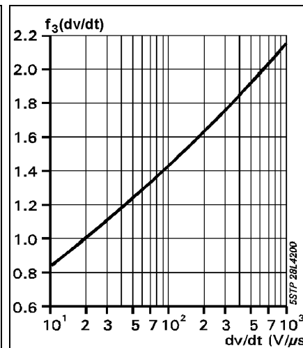
Fig. 14 t_q/t_{q1} = f_3(dv/dt)
