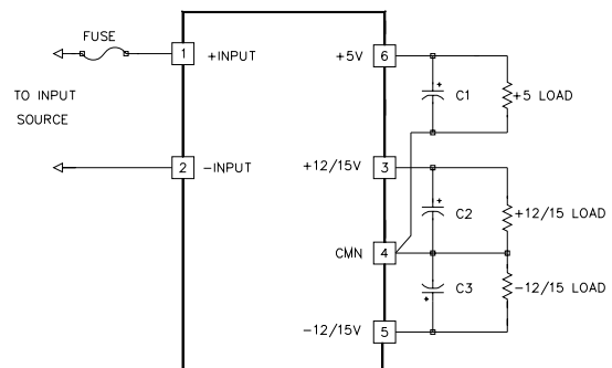
C1-C3=1µF/35V, TANTALUM
