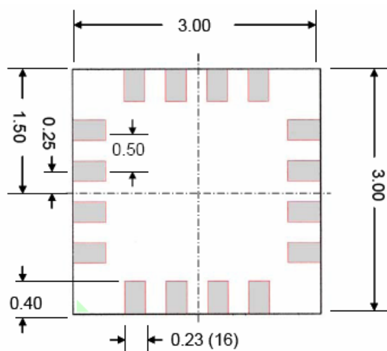
HMC1043 型底视图
