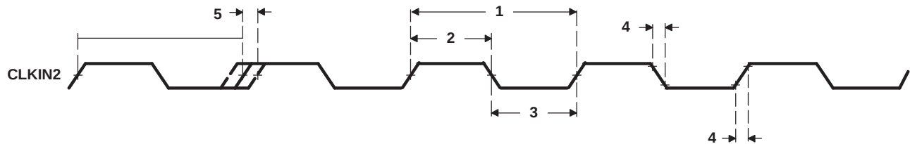
Figure 7-30. CLKIN2 Timing
