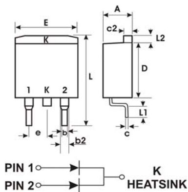
D 2 PAK
