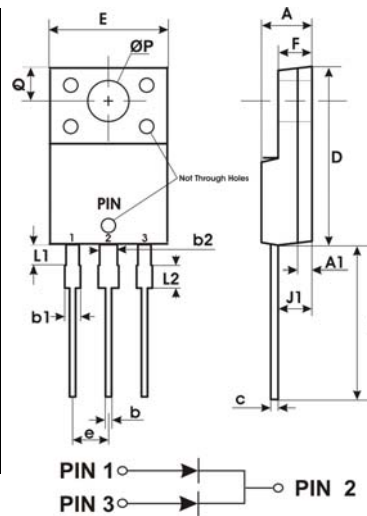
ITO-220AB
