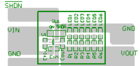
Fig. 16 Top-over layer
