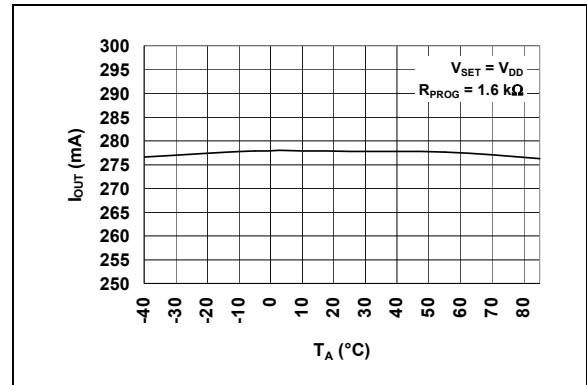
图 2-20: 充电电流 ( I_{OUT} ) 与环境温度 ( T_A ) 关系曲线
