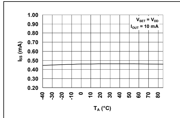
图 2-10: 电源电流 ( I_{SS} ) 与环境温度 ( T_A ) 关系曲线
