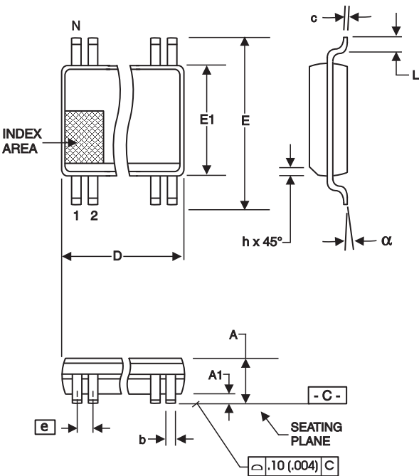
300 mil SSOP
