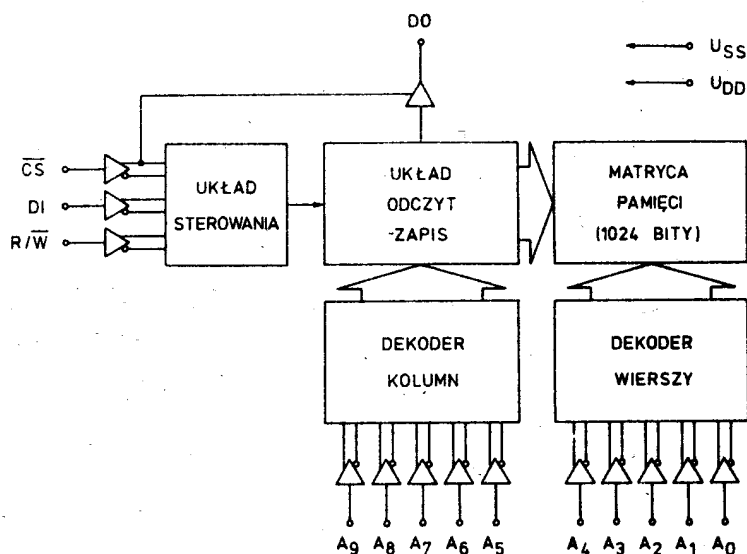
Blokowy schemat wewnętrzny
