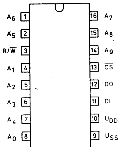
Układ wyprowadzeń
