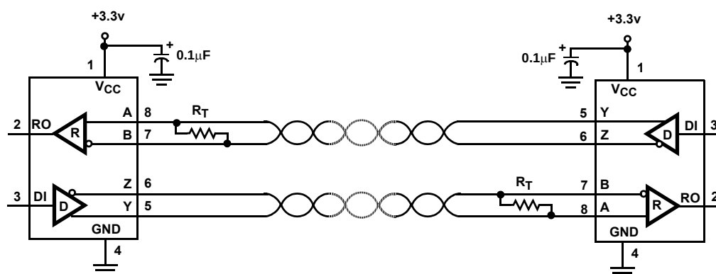
ISL83071E
