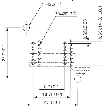
SSOP IC51-0302-755 (30 Pins)
