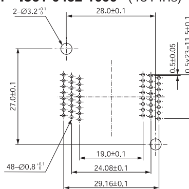
TSOP IC51-0482-2018 (48 Pins)
