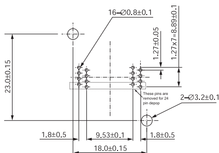
SOP IC51-347.KS-7704 (16 Pins)
