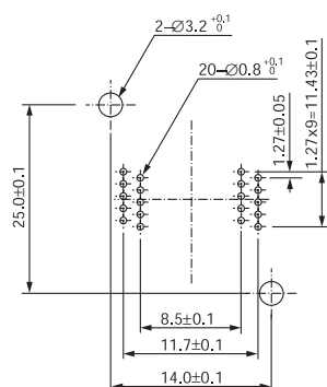
SOP IC51-0202-1026 (20 Pins)
