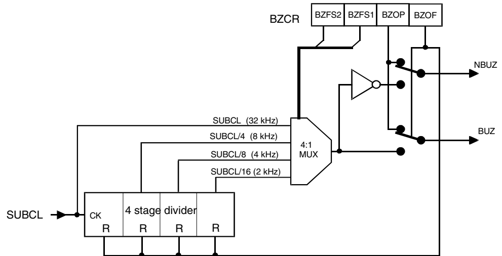
Figure 3-27. Buzzer Module
