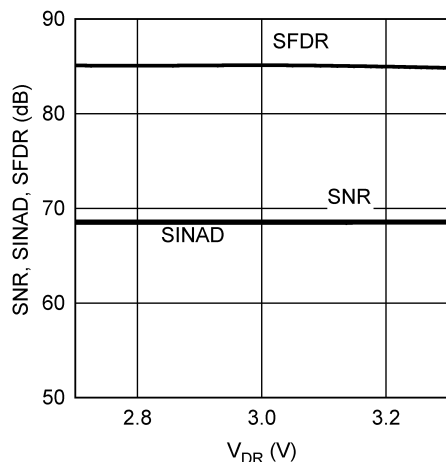
SNR, SINAD, SFDR vs. V_{DR} , V_A = V_D = 3.6V
