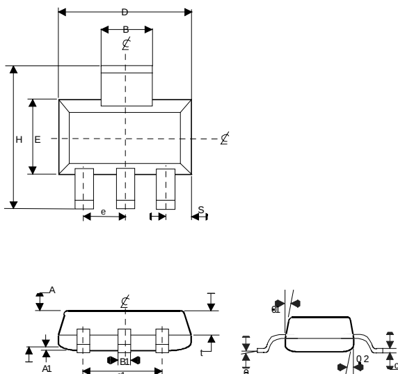
SOT 223
